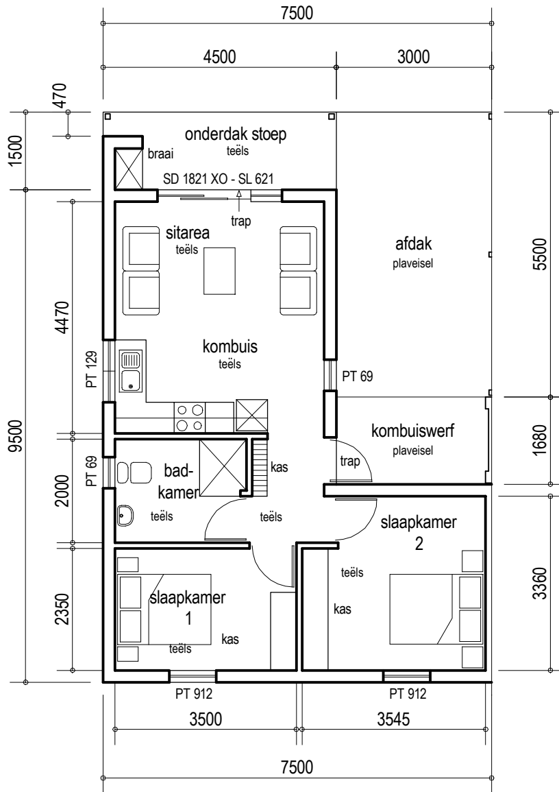
1:100 Grondvloerplan X77
