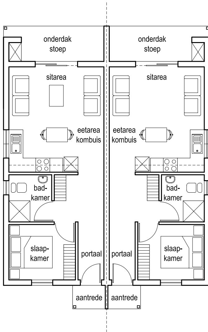
1:100 Grondvloerplan I50
